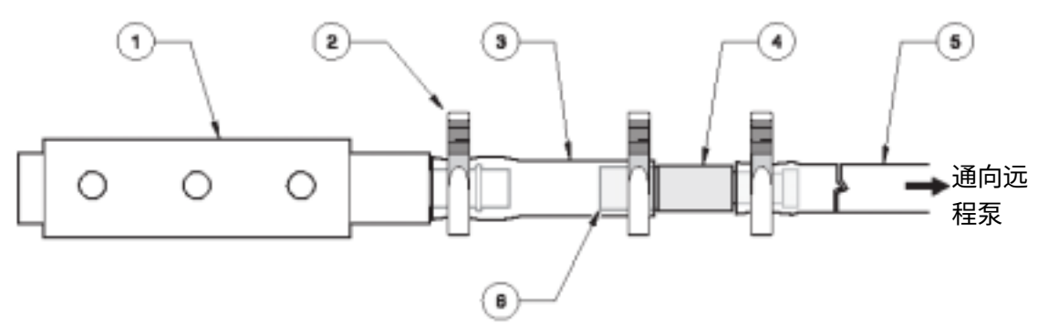
图 5 3/8 英寸内径管连到进口松紧扣和管接头
