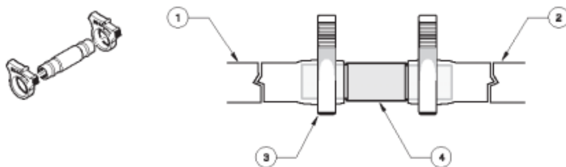
图 4 3/8 英寸乙烯管接到进口松紧扣和管接头
