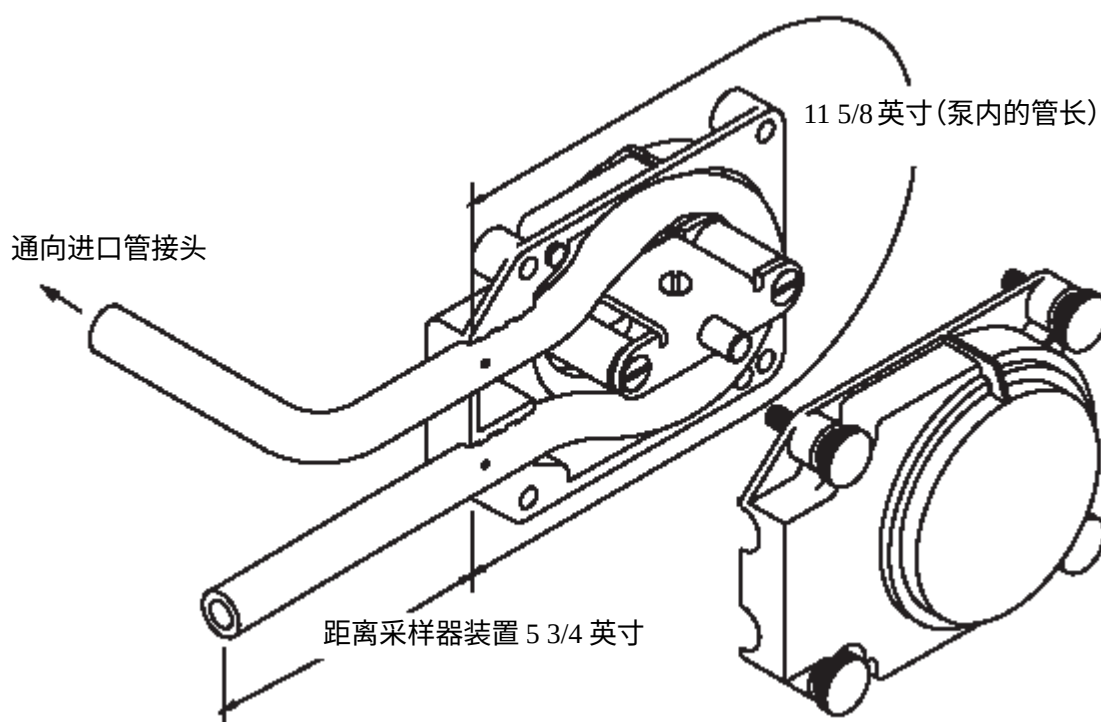
图 9 泵管安装
