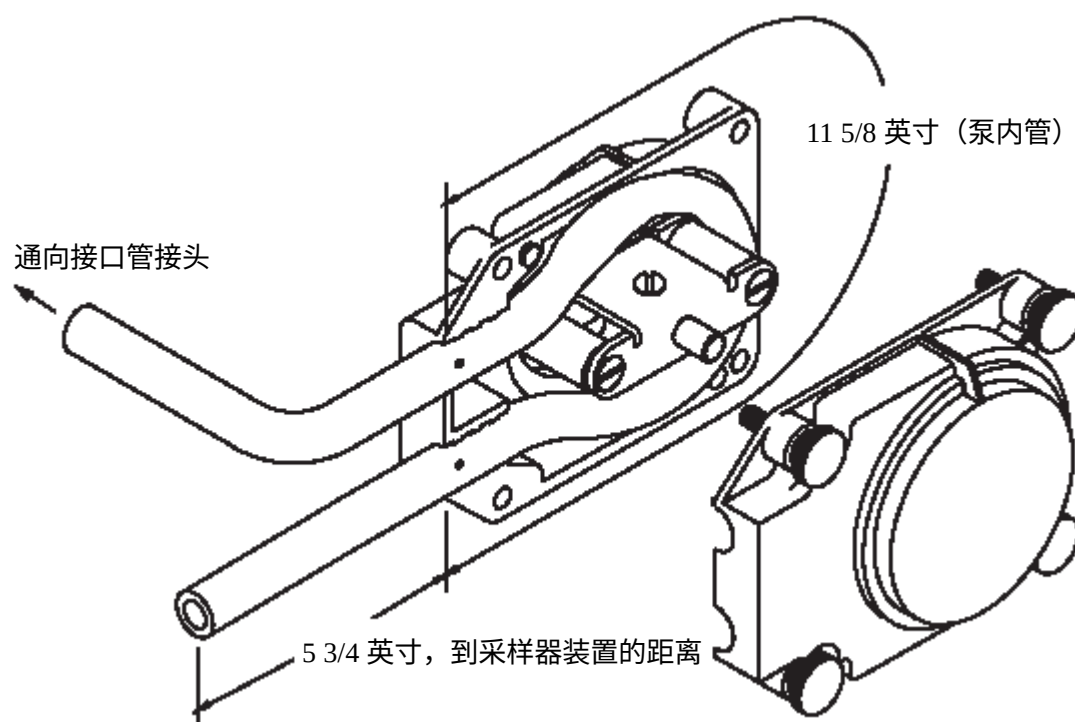
图 3 泵管的安装
